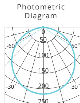
Unit: cd - C0/180 149.0deg - C90/270 113.7deg
